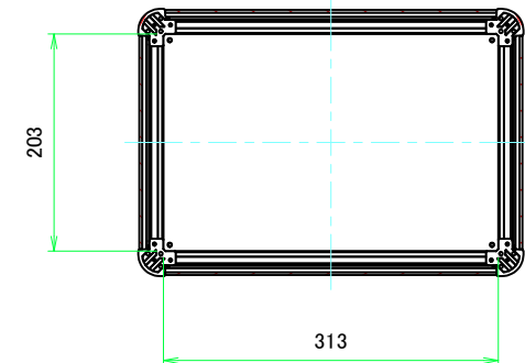
C-C (1 : 5.5)
